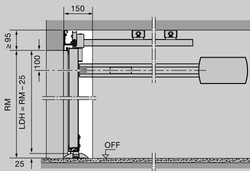
Montage mural de la motorisation
