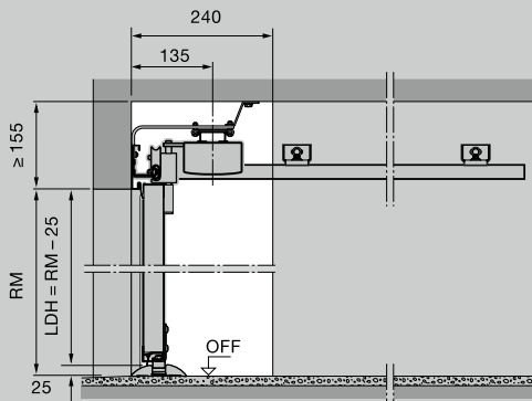
Montage au plafond de la motorisation
