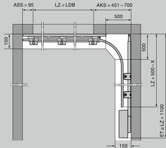
Ferrure ES (rail simple - montage mural de la motorisation)
