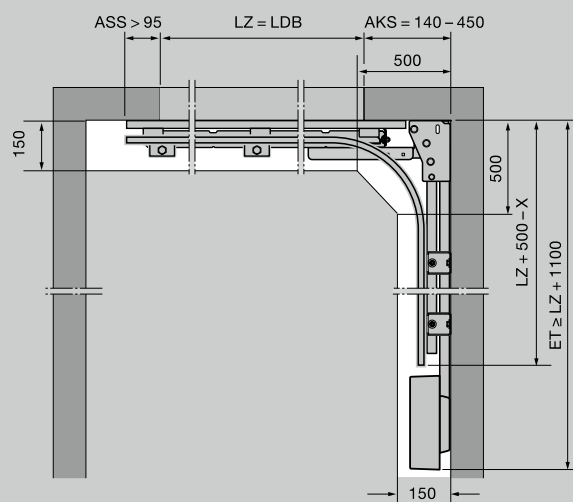
Ferrure DS (rail double - montage mural de la motorisation)
