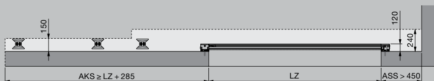
Montage au plafond B en tant que porte coulissante (coupe du rail de sol)
