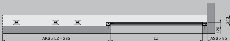
Montage mural en tant que porte coulissante (coupe du rail de sol)
