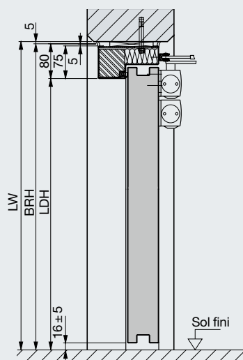
Coupe verticale
