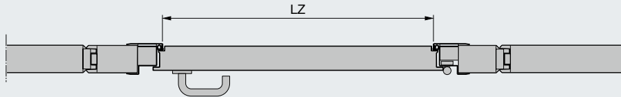
Coupe horizontale
