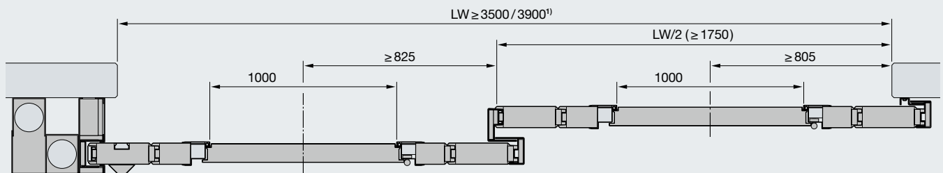
Partie poignée
