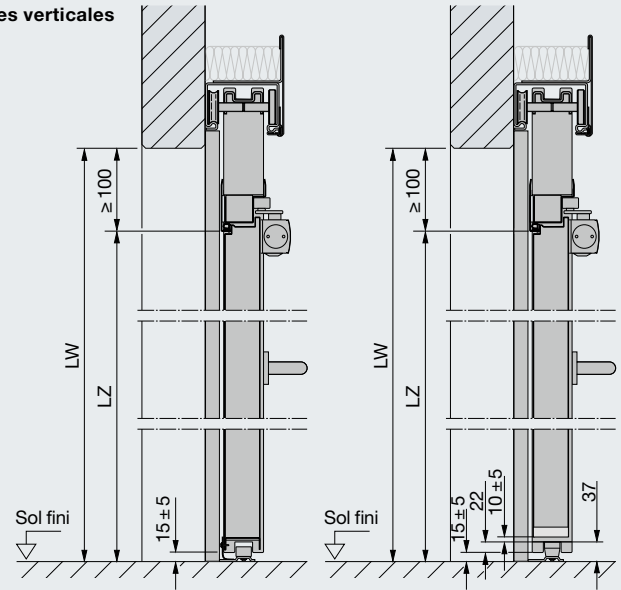
Porte de passage avec seuil de 22 mm
